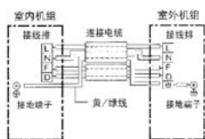
图14 室内外电气连接图
